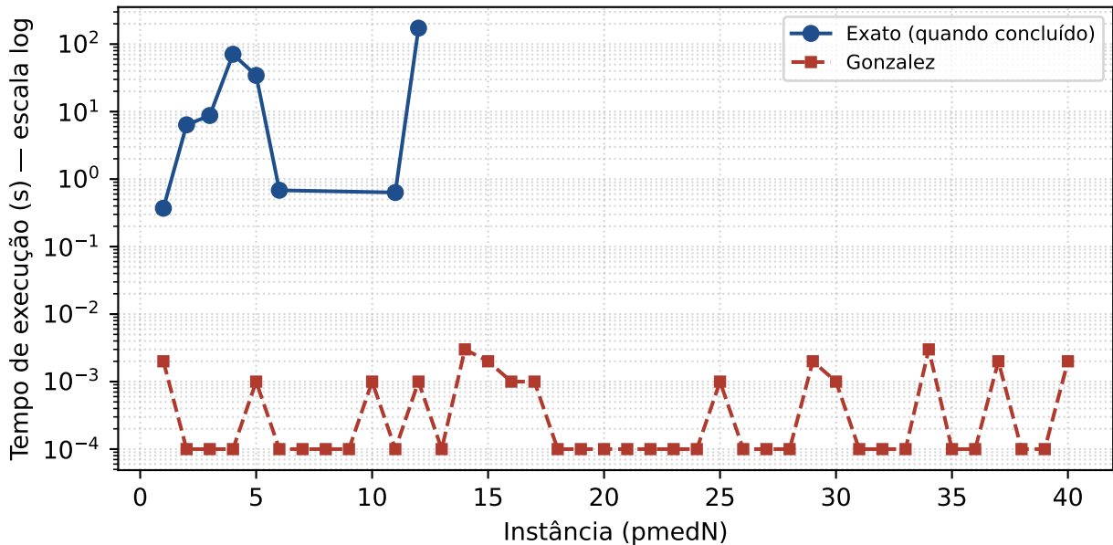
Tempo de execução: Exato vs. Gonzalez
